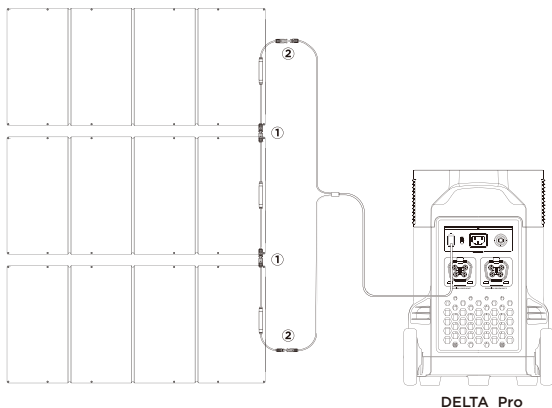
DELTA Pro
